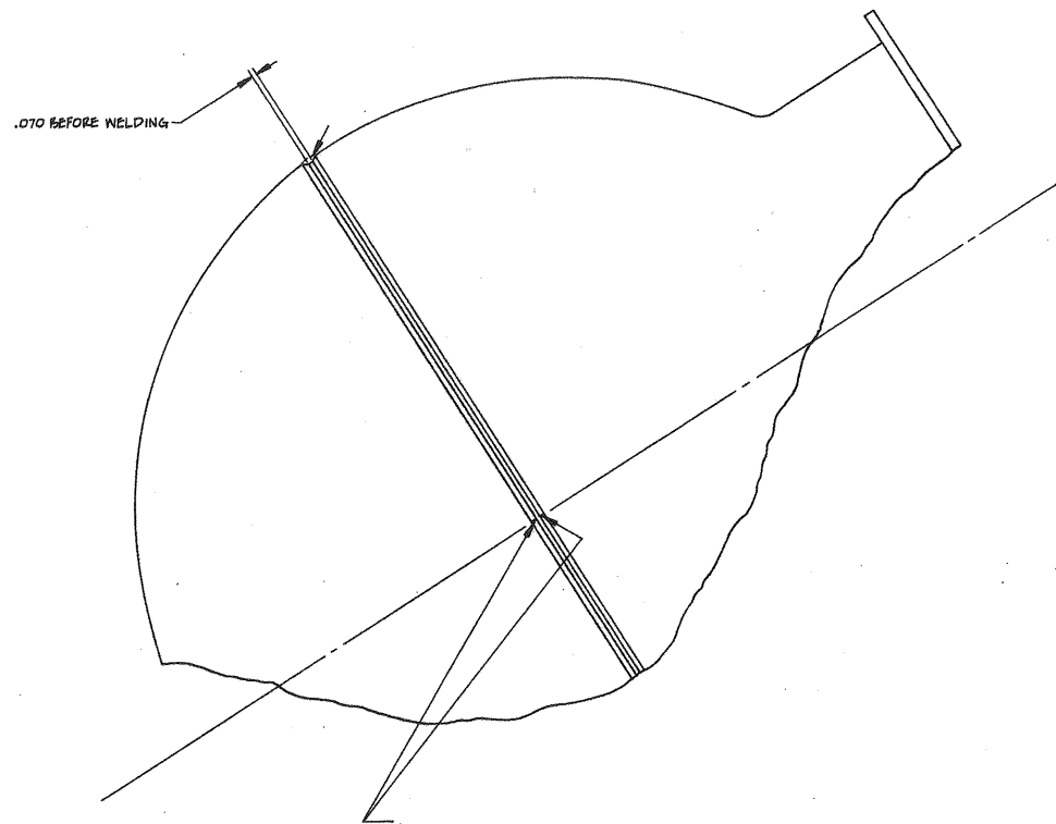
VIEW A-A
