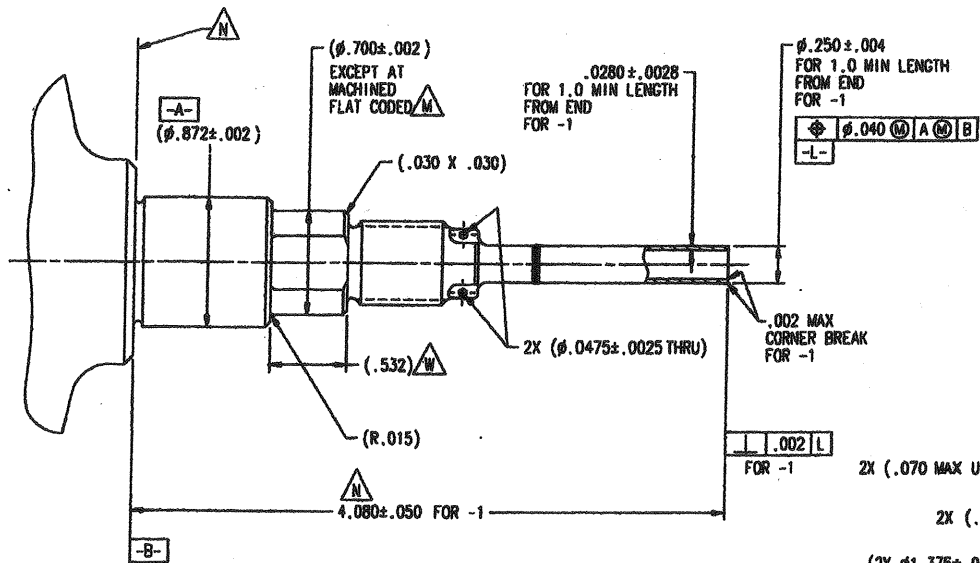
VIEW H SCALE: 2/1
