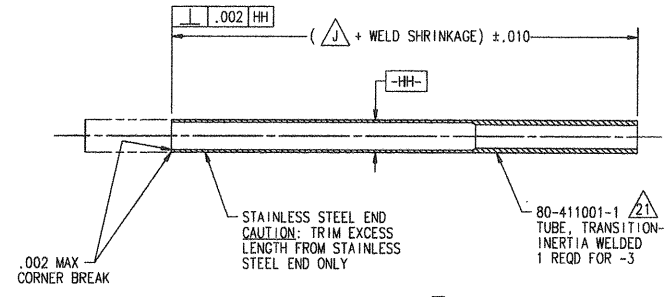
DETAIL -3 SCALE: 2/1
