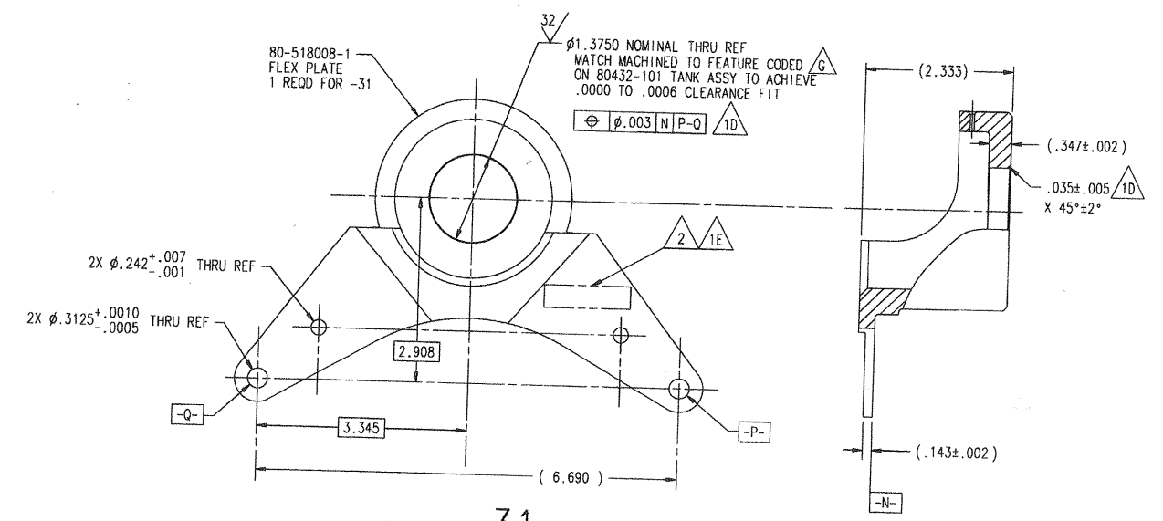
DETAIL -31 SCALE: 1/1
