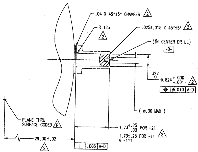
VIEW B SCALE: 1/1
