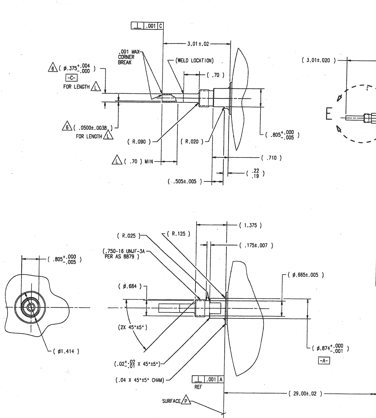
VIEW E SCALE: 1/1
