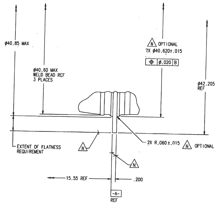
VIEW F SHEET 1 SCALE: 1/1
